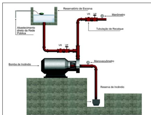
VR - Válvula de retenção VP - Válvula de paragem
