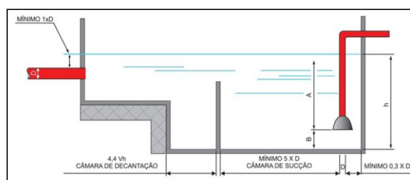
Figura B.6 - Alimentação natural de reservatório por conduto
