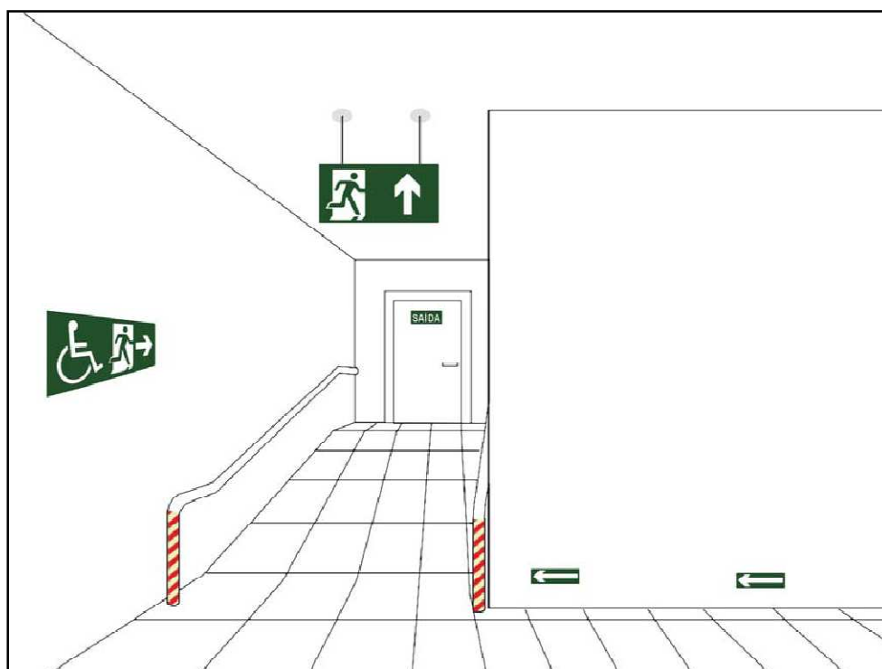
Figura C-15: Sinalização de saída em rampa
