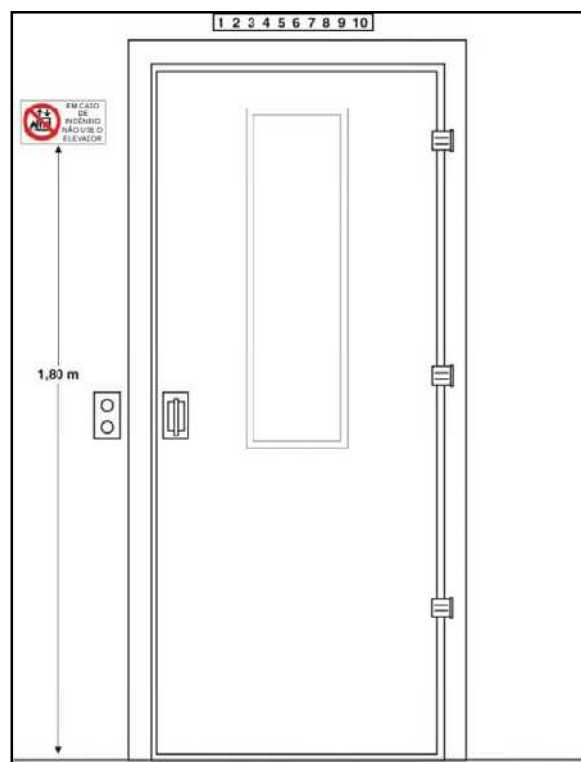
Figura C-4: Sinalização de elevadores (vista da escada)
