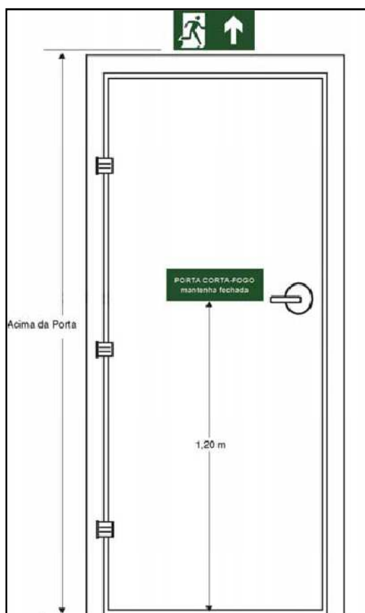
Figura C-1: Sinalização de porta corta-fogo (vista da escada)
