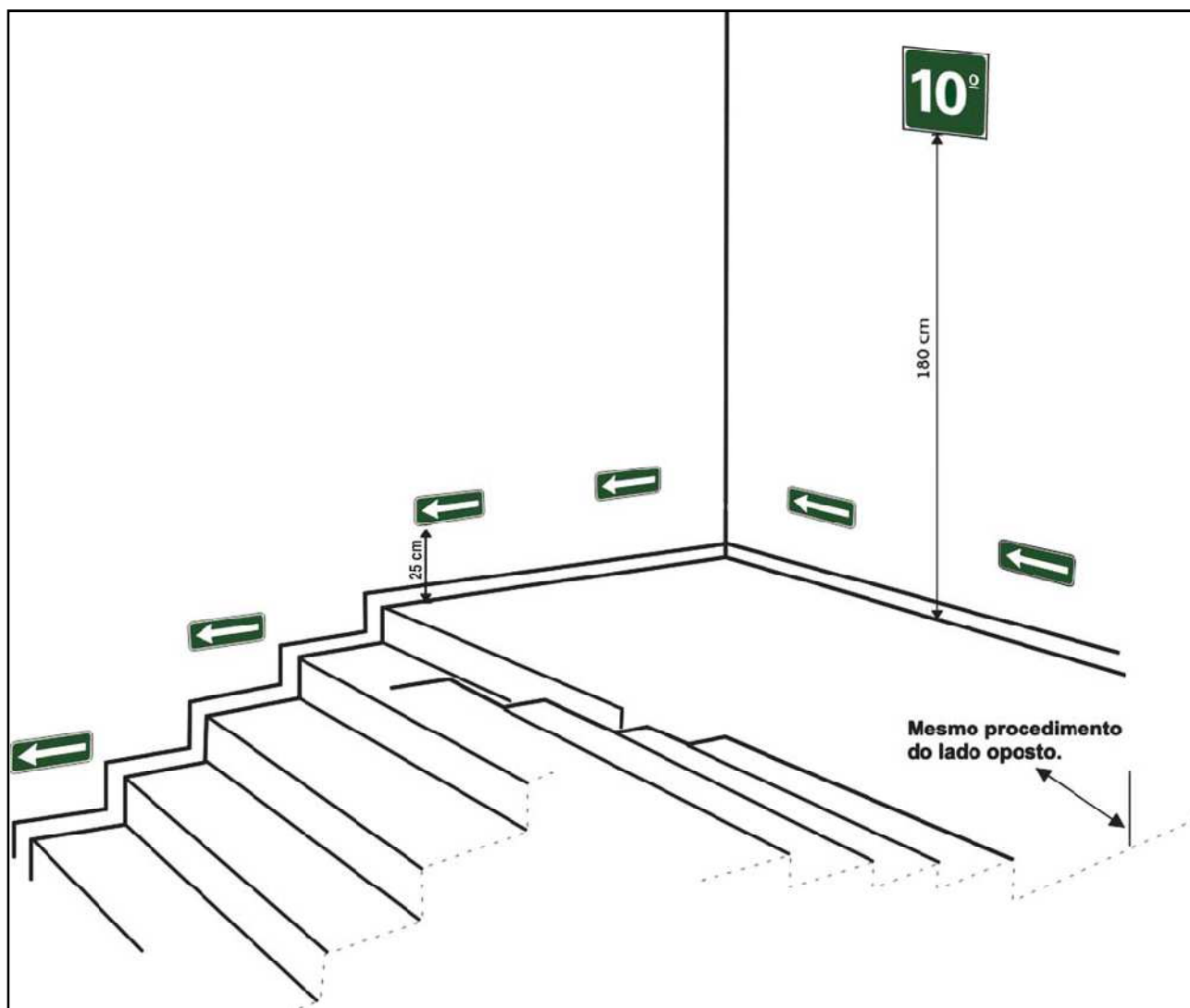
Figura C-8: Sinalização complementar. Exemplo de rodapé
