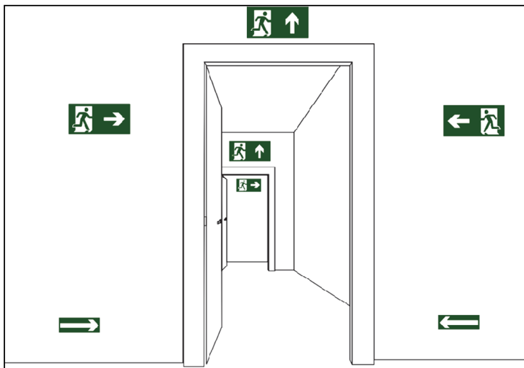
Figura C-11: Sinalização de saída sobre paredes e vergas de portas
