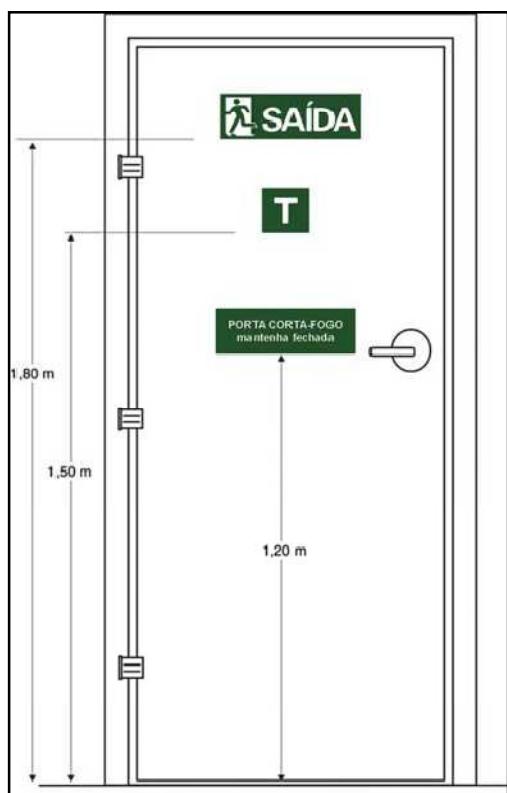
Figura C-3: Sinalização de porta corta-fogo
