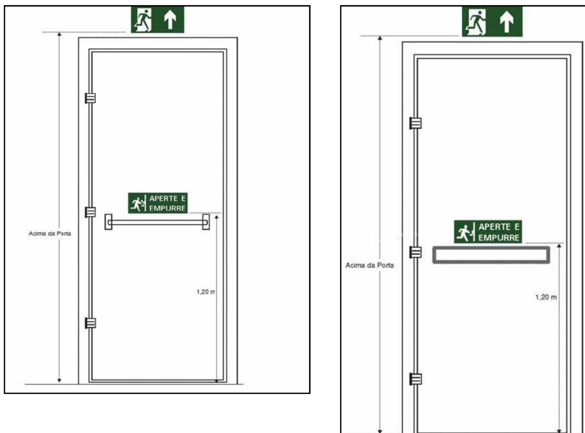
Figura C-5: Sinalização de portas com barras antipânico (modelos 1 e 2)
