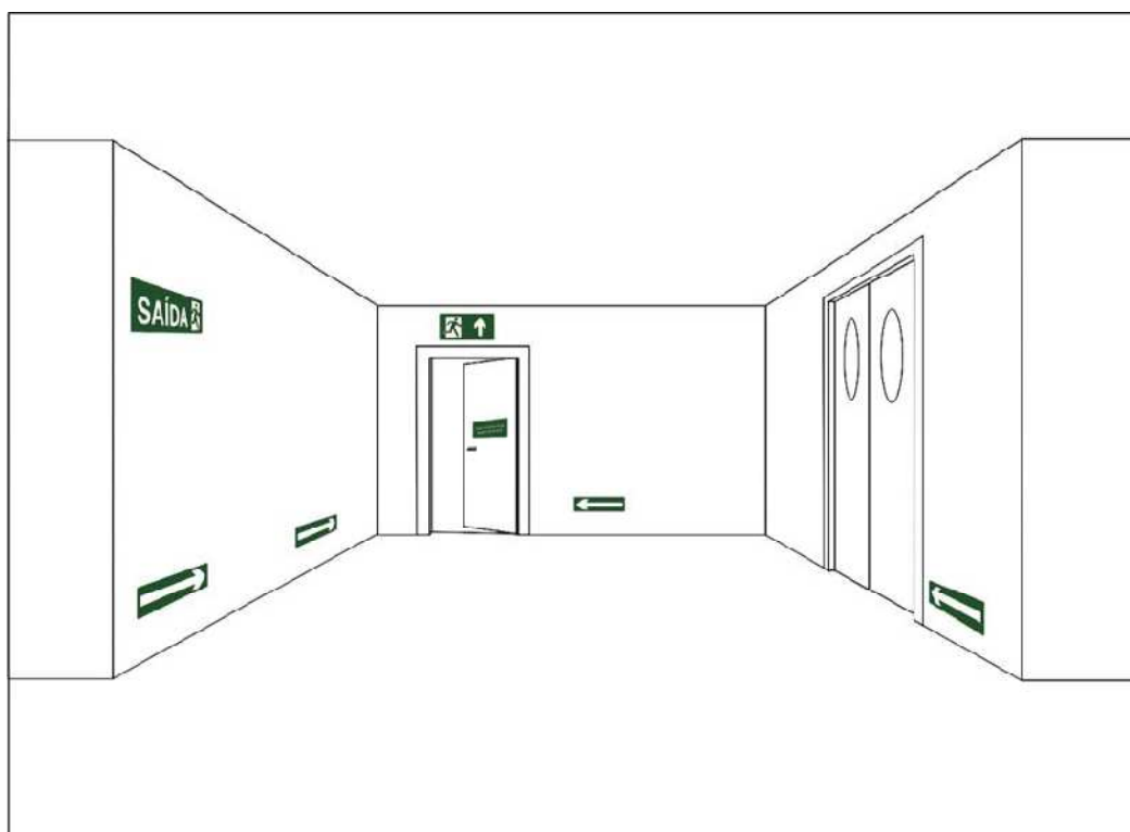
Figura C-12: Sinalização de saída sobre porta corta-fogo
