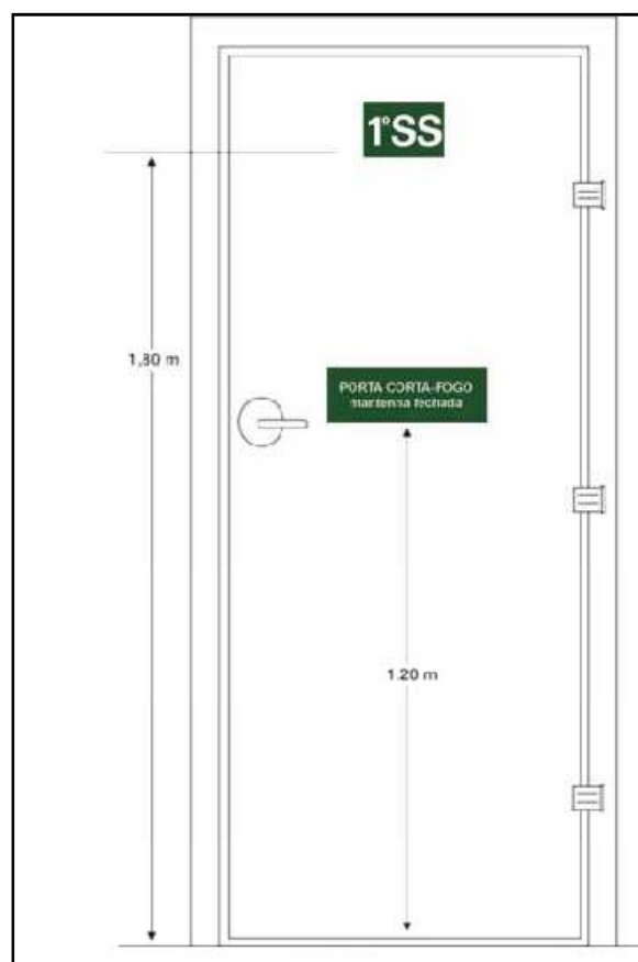
Figura C-2: Sinalização de porta corta-fogo (vista do hall)
