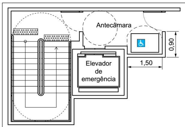
Figura 9b: Escada com representação da área de resgate para pessoas com deficiência
