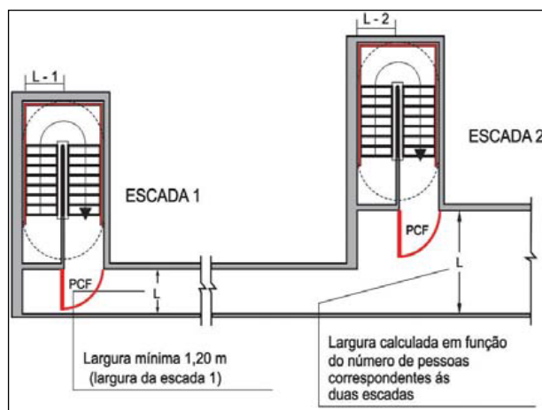
Figura 18: Dimensionamento de corredores de descarga
