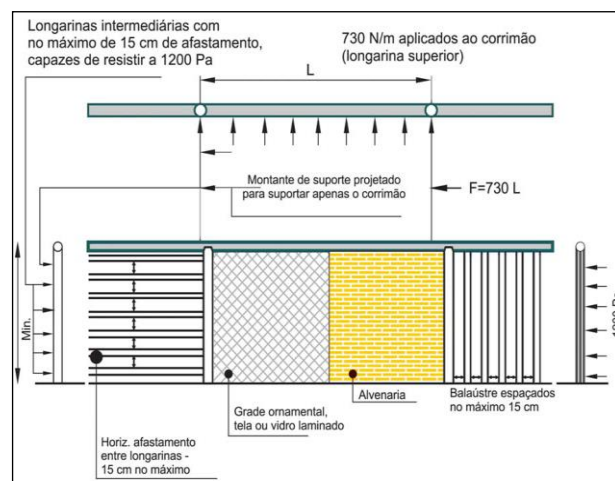
Figura 16: Pormenores construtivos da instalação de guardas e as cargas a que elas devem resistir
