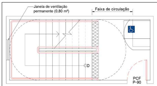
Figura 7a: Escada enclausurada protegida
