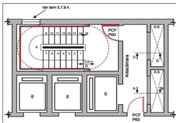
Figura 9a: Escada enclausurada à prova de fumaça com representação dos dutos de entrada e saída de ar
