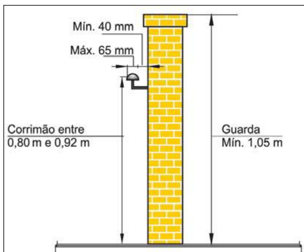
Figura 14: Dimensões de guardas e corrimãos
