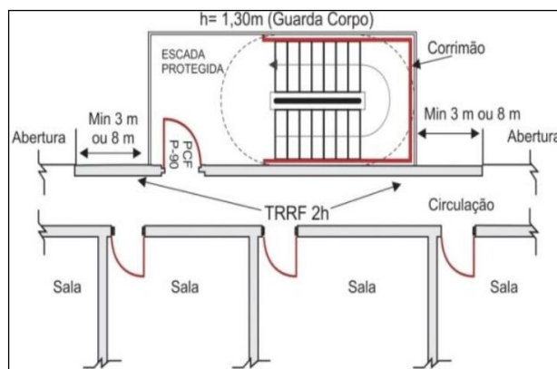
Figura 12: Escada aberta externa
