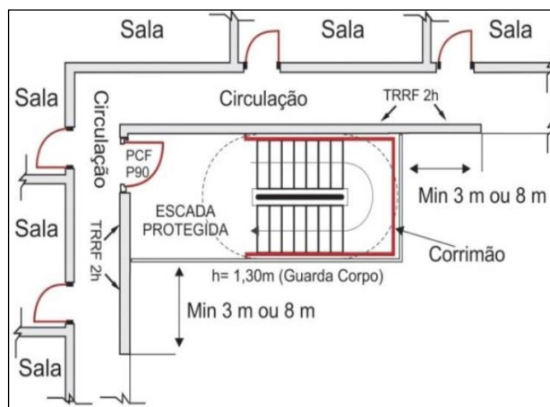
Figura 13: Escada aberta externa
