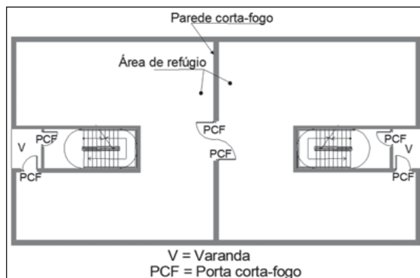
Figura 17: Desenho esquemático da área de refúgio
