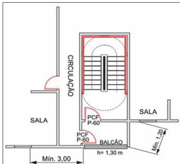
Figura 11: Escada enclausurada do tipo PF ventilada por balcão
