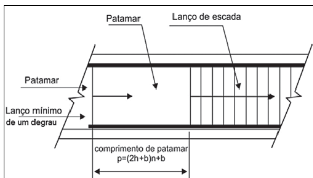
Figura 6: Lanço mínimo e comprimento de patamar
