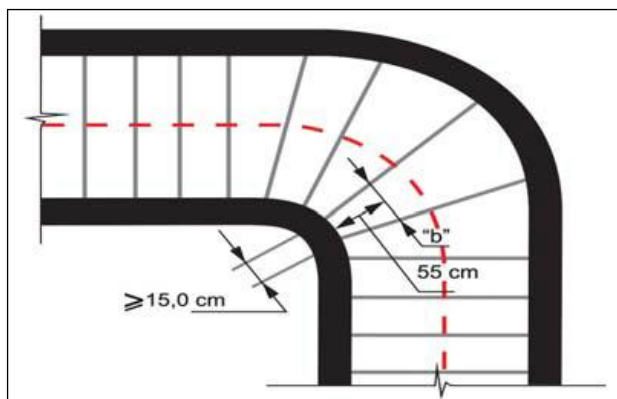
Figura 5: Escada com lanços curvos e degraus balanceados
