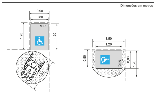
Figura 7b: Espaço para PCR realizar movimentação em locais confinados
