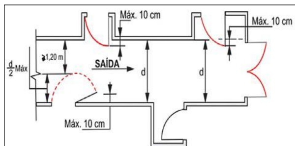
Figura 2: Abertura das portas no sentido de saída
